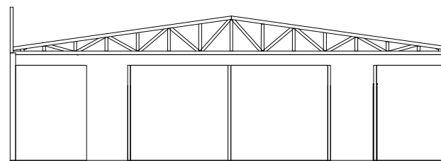
4 Corte A 1 : 50
