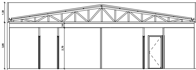
2 Corte C 1 : 50
